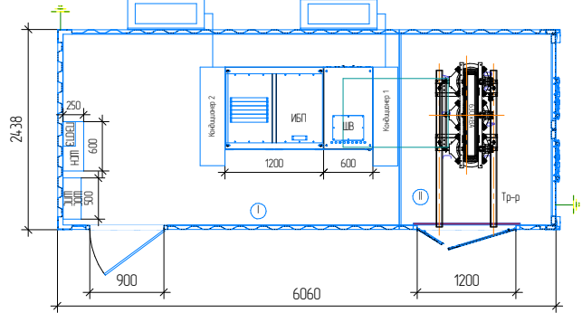
План размещения оборудования АКБ. М140.
